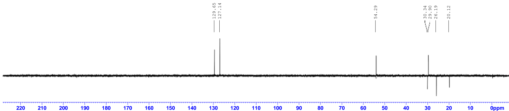
13C{1H}com AV500
