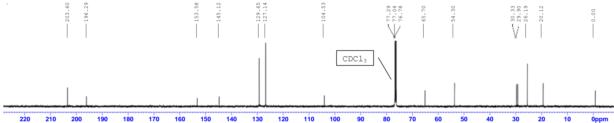
13C{1H}com AV500
